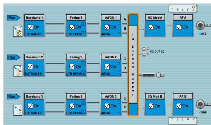
Блок-схема генератора R&S®SMW200A, настроенного на формирование тестового сценария LTE Release 11 feICIC. Один генератор R&S®SMW200A одновременно формирует сигналы обслуживающей соты LTE, а также двух мешающих сот; для каждой соты реализована схема MIMO 2x2 с коррелированными каналами замираний.
