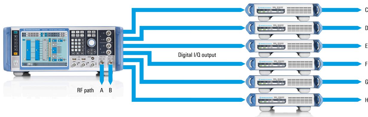
Система 4x8 MIMO, состоящая из двухканального генератора сигналов R&S®SMW200A и шести модулей генерации сигналов R&S®SGT100A, управляемых с генератора R&S®SMW200A. Модули реализуют ВЧ-тракты с 3 по 8. Генератор R&S®SMW200A обеспечивает полноценное формирование модулирующего сигнала и имитацию замираний.
